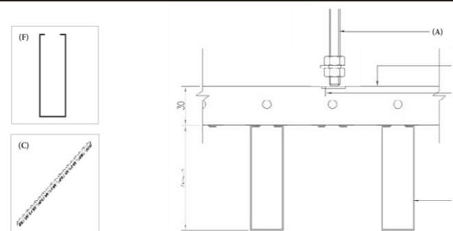
Section Drawing / 正面节点图
