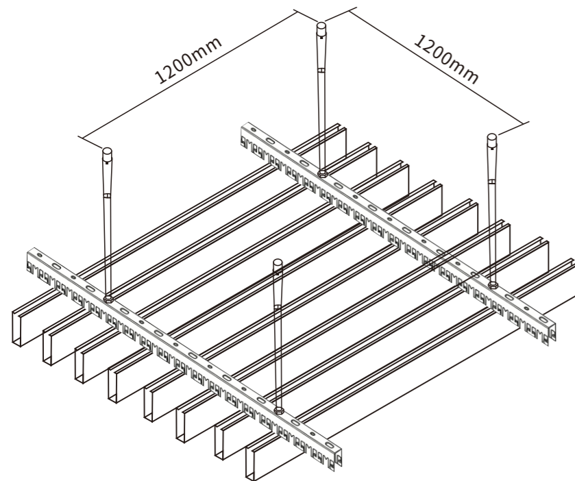
(INSTALLATION DIAGRAM) 安装示意图
